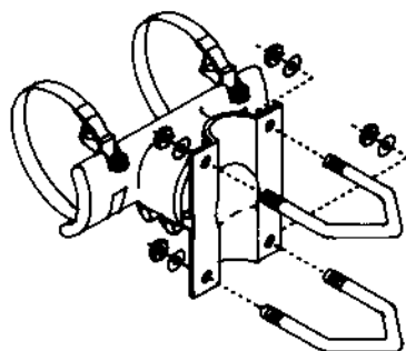
"E" (PELCO AB-3004)
